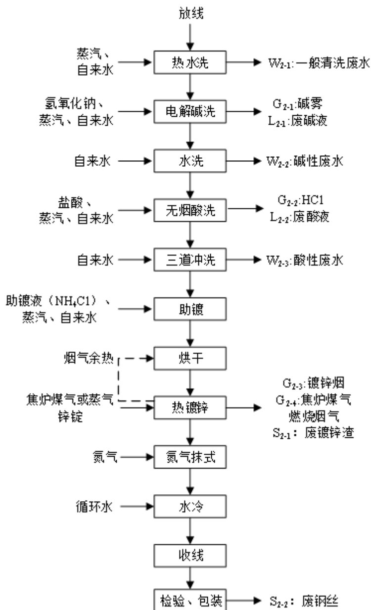
图 2.4-6 热镀锌钢丝工艺流程及产污环节图
