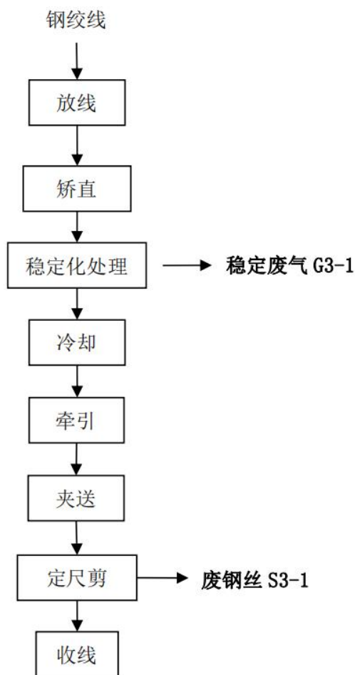
图 2.4-3 低松弛预应力钢丝工艺流程及产污环节图
