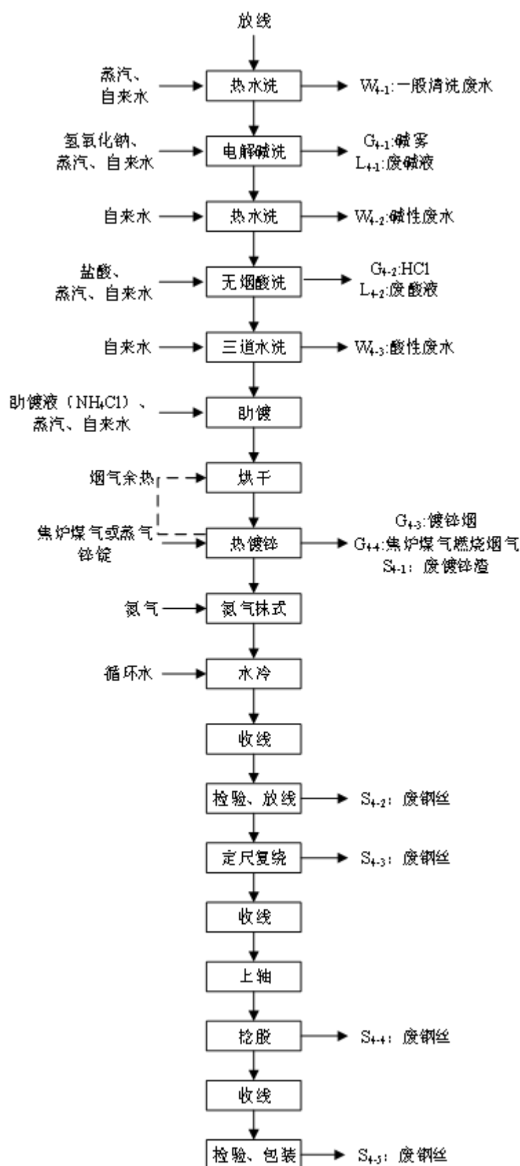
图 2.4-7 热镀锌钢绞线工艺流程及产污环节图
