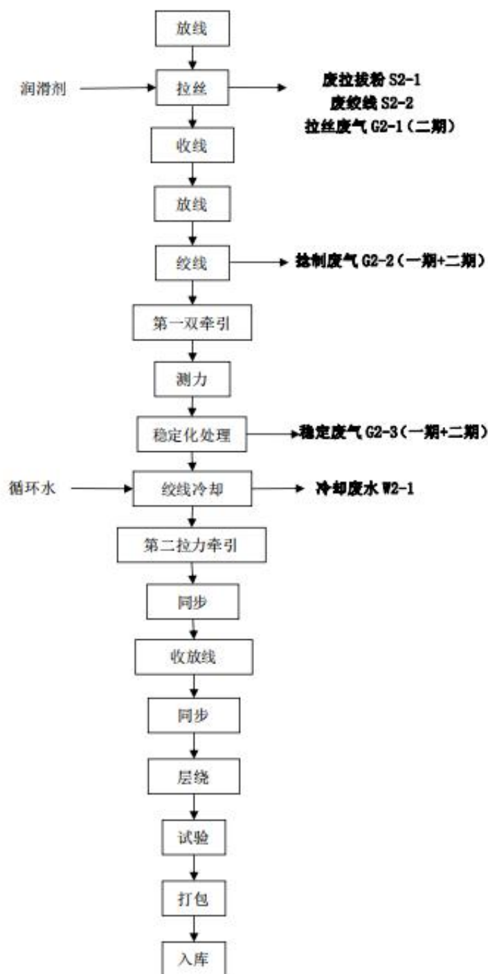
图 2.4-2 低松弛预应力钢绞线工艺流程及产污环节图
