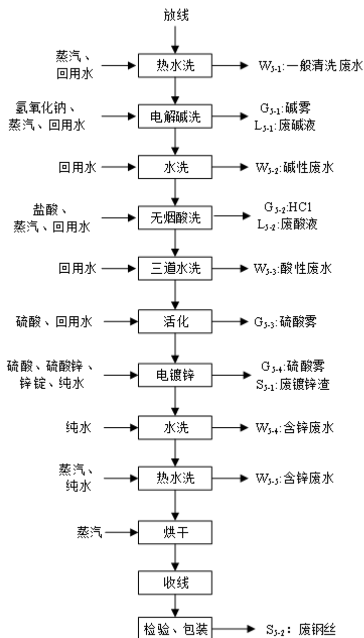
图 2.4-8 电镀锌钢丝工艺流程及产污环节图
