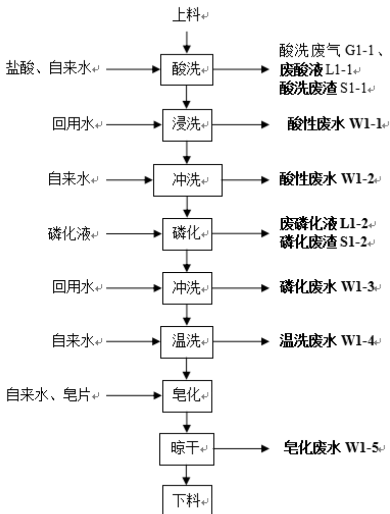
图 2.4-1 酸洗车间工艺流程及产污环节
