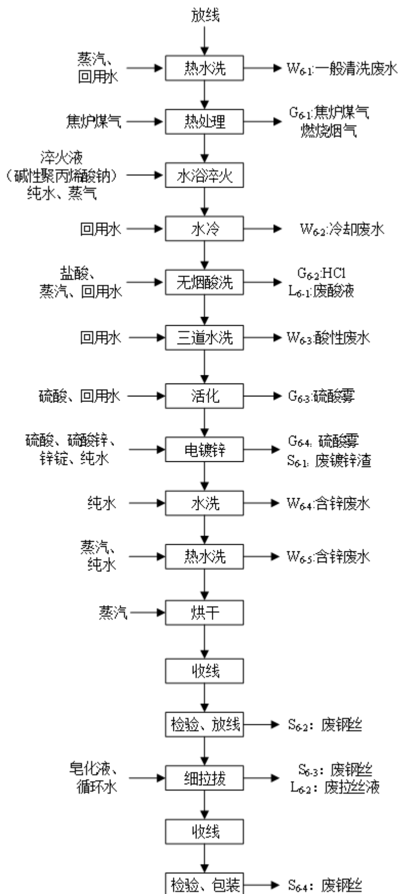
图 2.4-9 细直径电镀锌钢丝工艺流程及产污环节图
