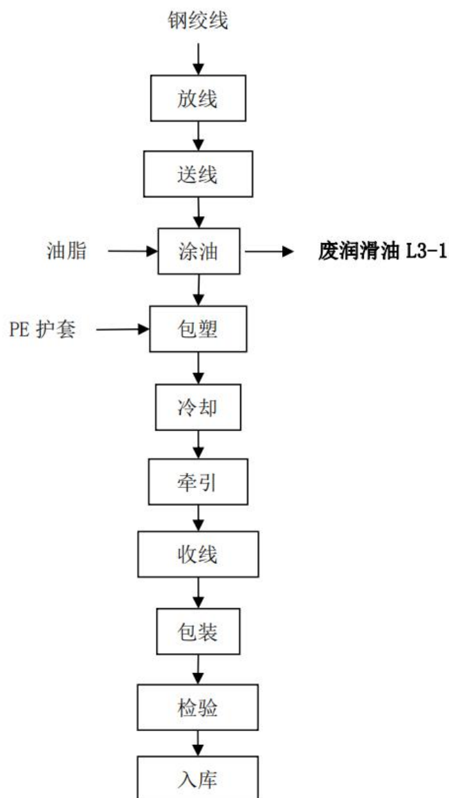
图 2.4-4 无粘结预应力钢绞线工艺流程及产污环节图
