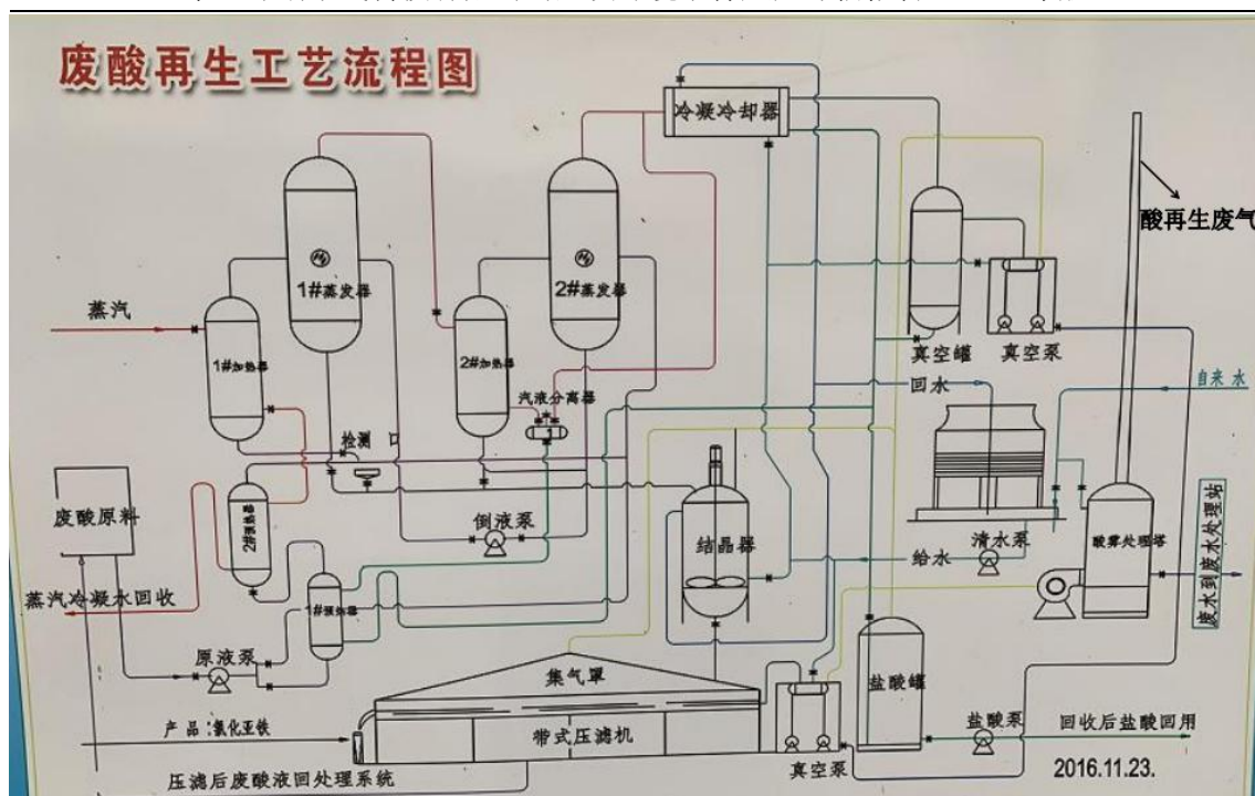
图 2.4-5 酸再生系统工艺流程及产污环节图
